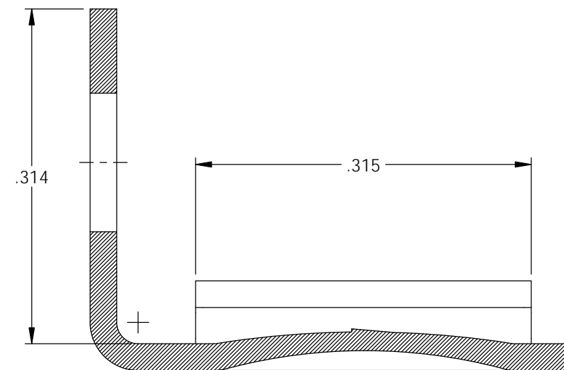
SECTION A-A
