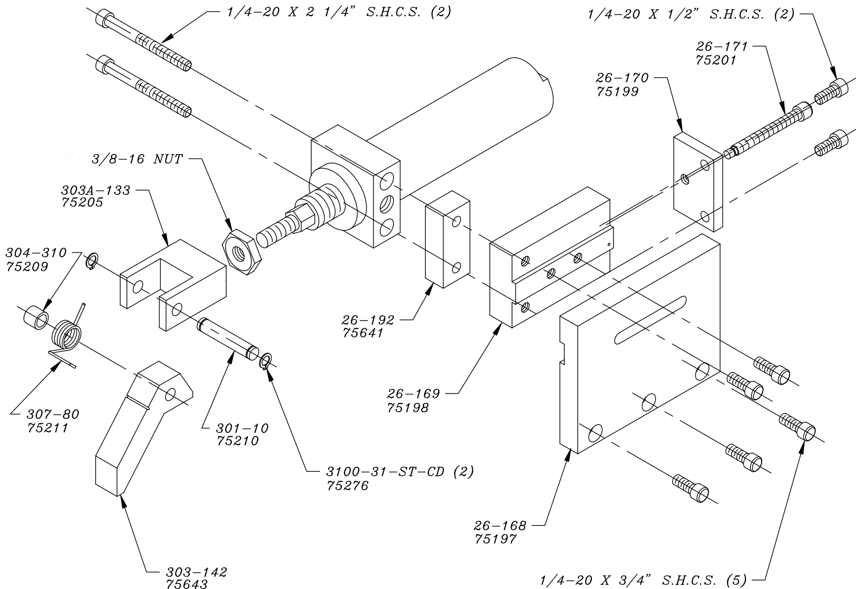
DIE SET APPLICATOR HMD 82330
