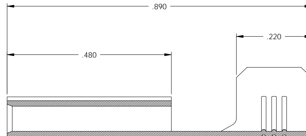
SECTION A-A SCALE 6 : 1
