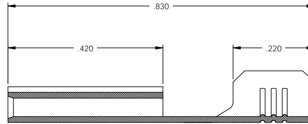
SECTION A-A SCALE 6 : 1
