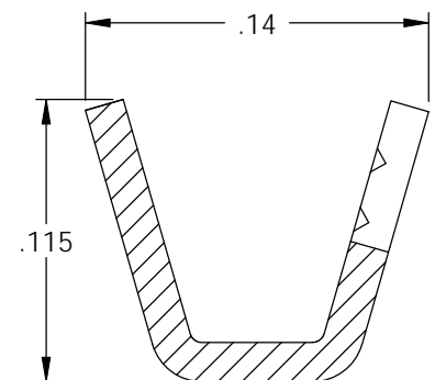
SECTION B-B SCALE 12 : 1
